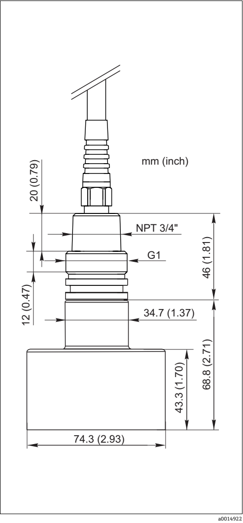
标准传感器的外形尺寸示意图
