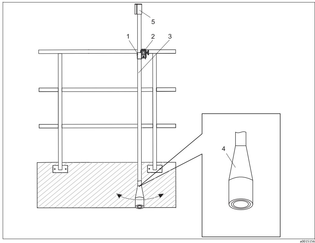
测量系统示意图，带悬挂支座
