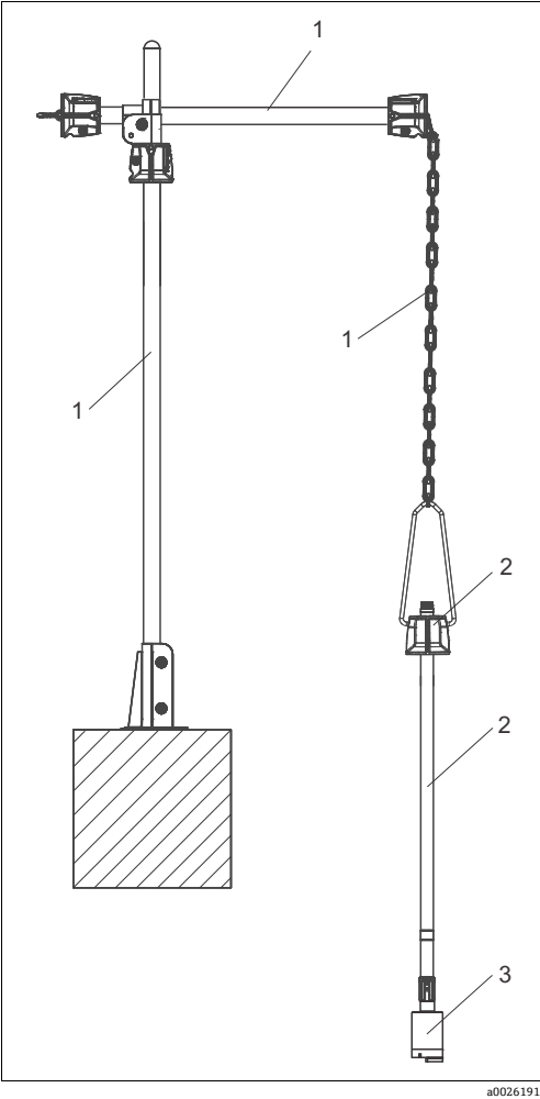
测量系统示意图，带链条式安装支座
