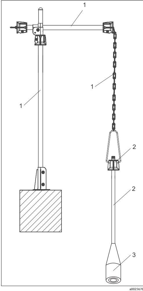
测量系统示意图，带链条式安装支座
