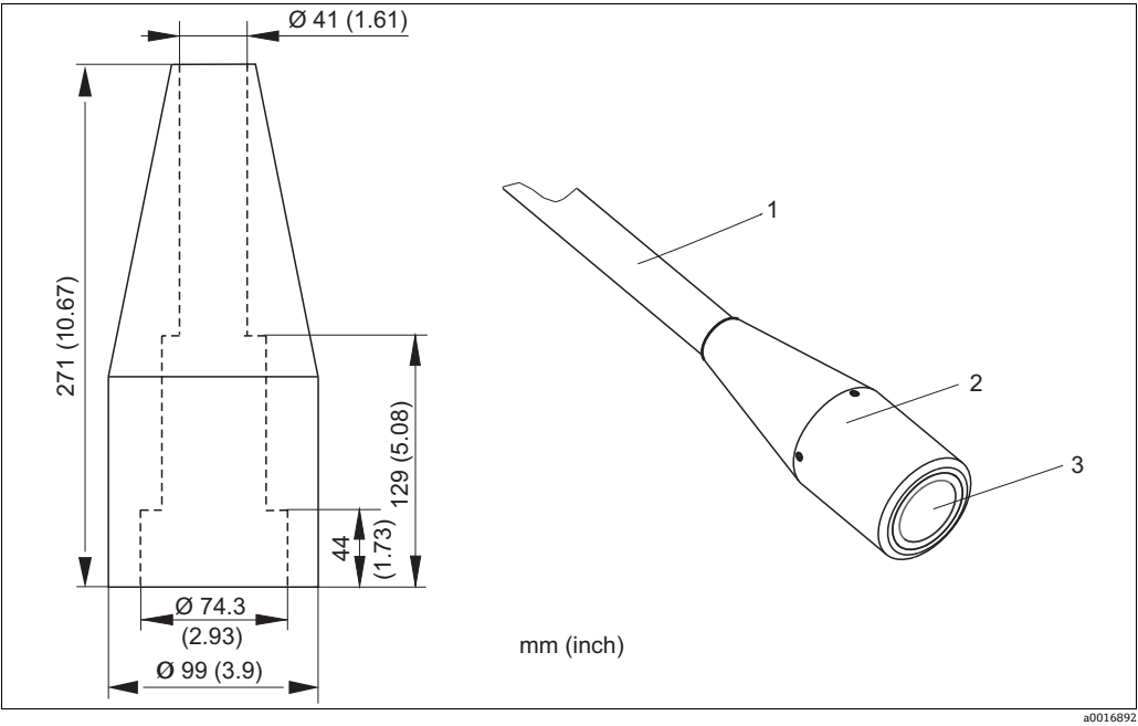
CUS71D 的 PVC 传感器保护头 1 CYA112 安装支架 2 PVC 保护头 3 CUS71D 超声波污泥界面传感器
