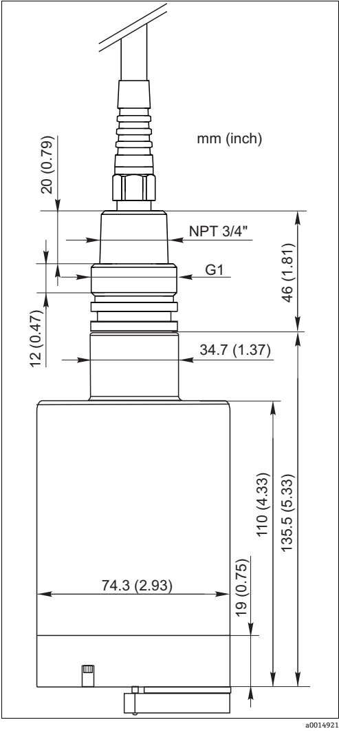
带刮刷的传感器的外形尺寸示意图
