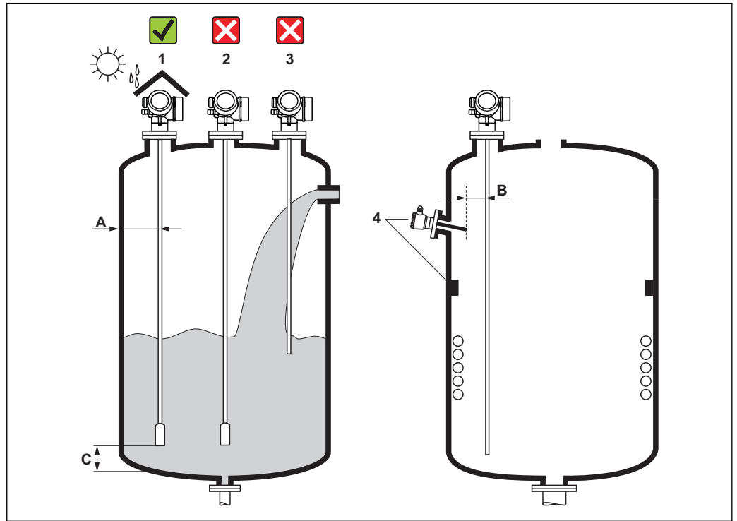
图 8 Levelflex 的安装要求
