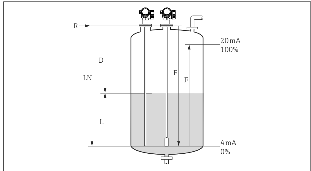
图 1 导波雷达的料位测量参数
