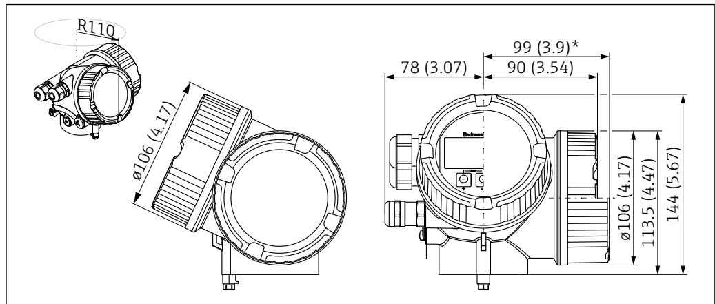
图 14 GT19 外壳 (塑料 PBT) ; 单位: mm (in)
