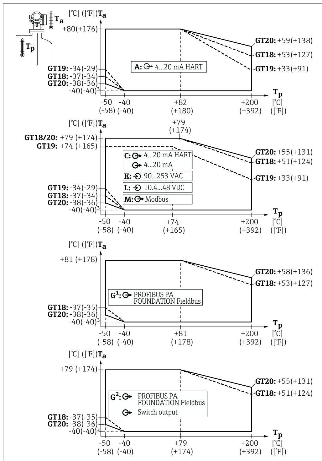
温度曲线: FMP51, 带法兰连接
