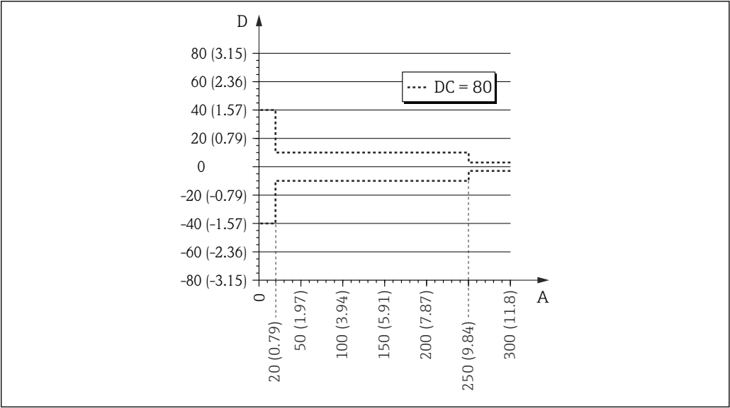
5 缆式探头底部附近的测量误差
