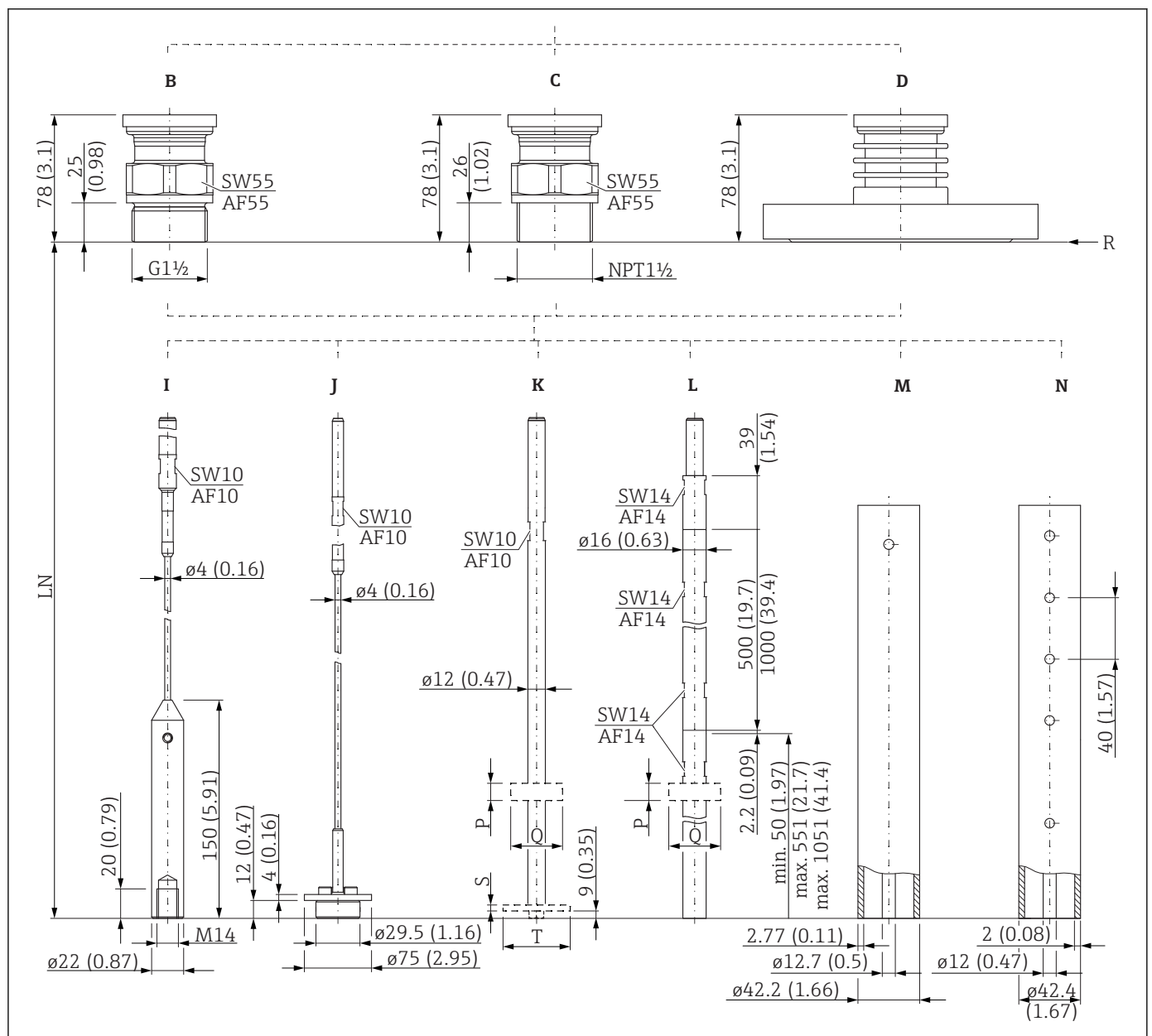
图 19 FMP51 的过程连接 / 探头; 单位: mm (in)。测量单位 mm (in)
