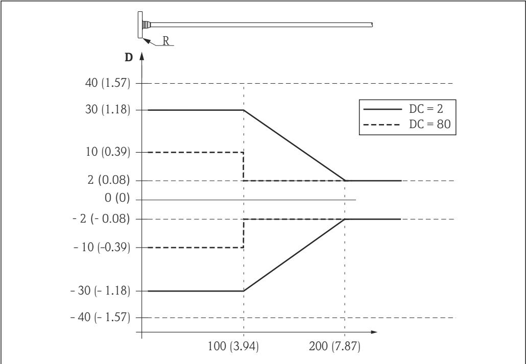
图 7 缆式探头顶部附近的测量误差；单位：mm (in)
