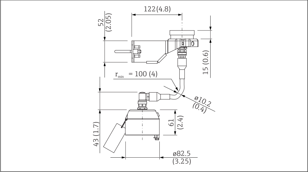
17 分体式探头的连接尺寸；单位：mm (in)；连接电缆长度为订购长度
