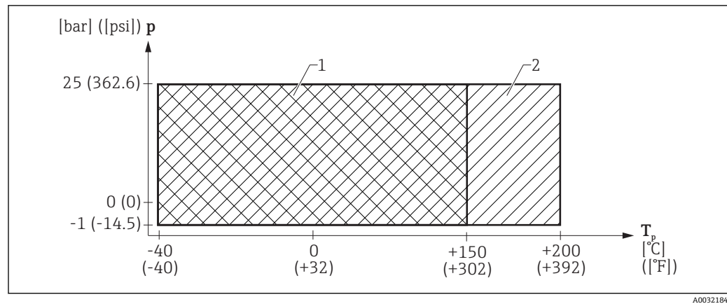
图 17 FMR62: 允许过程温度和过程压力范围, 带法兰或 DIN11851 过程连接
