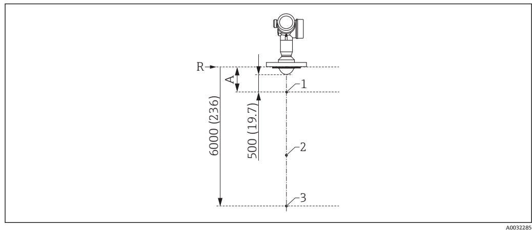
图 33 三点线性标定中的三个标定点的图示说明; 单位: mm (in)
