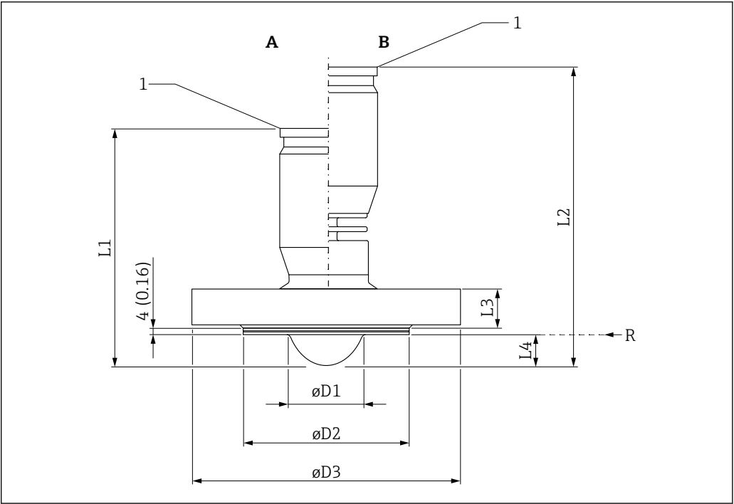
25 外形尺寸示意图; 单位: mm (in)
