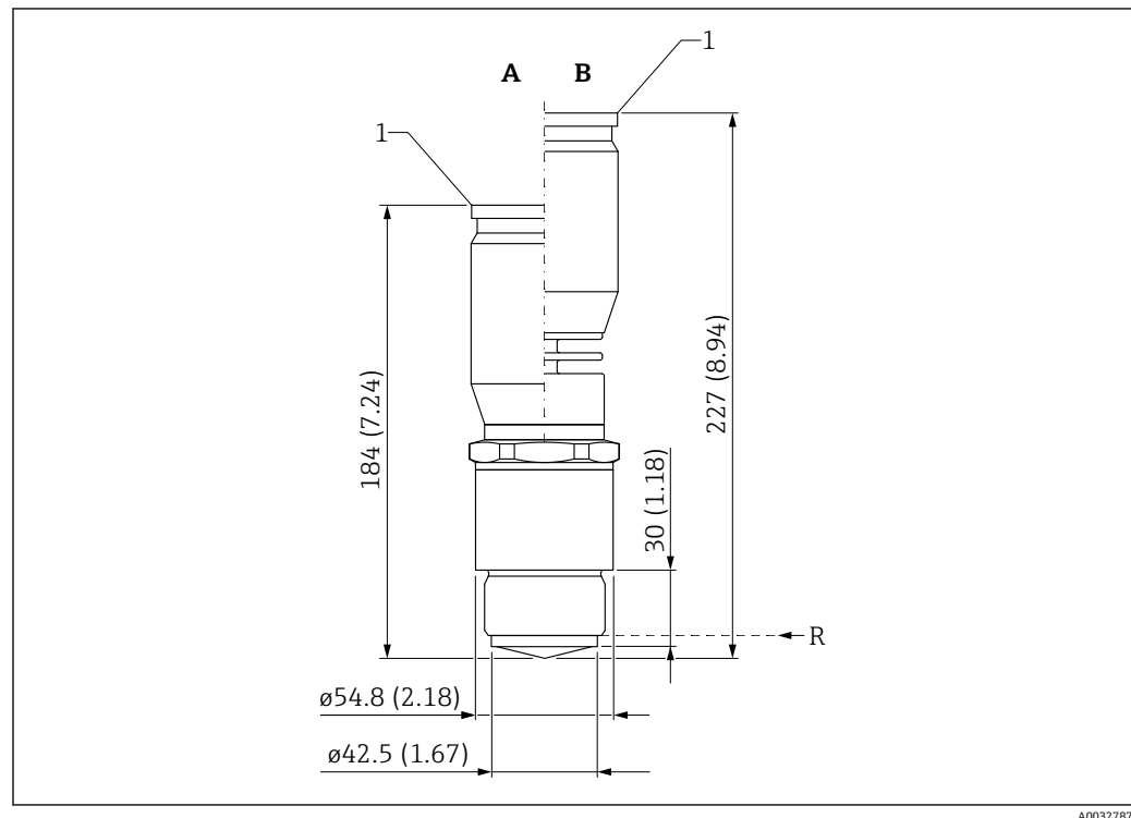
图 22 外形尺寸示意图; 单位: mm (in)
