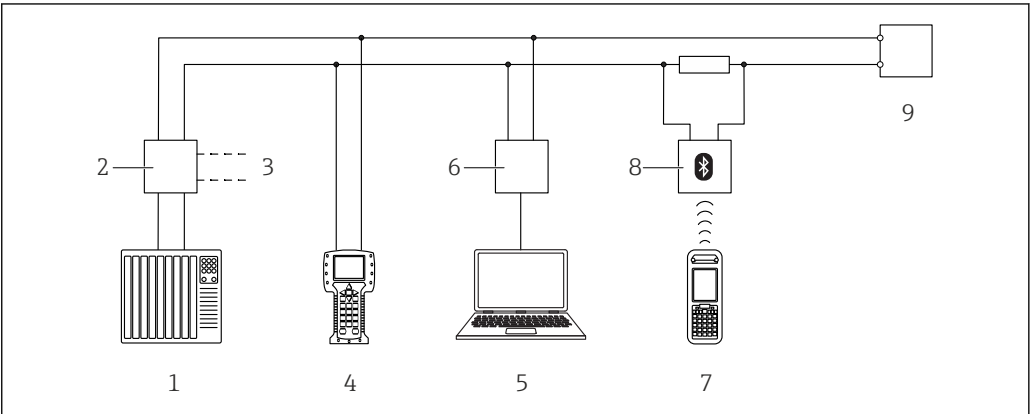
29 通过 HART 通信进行远程操作
