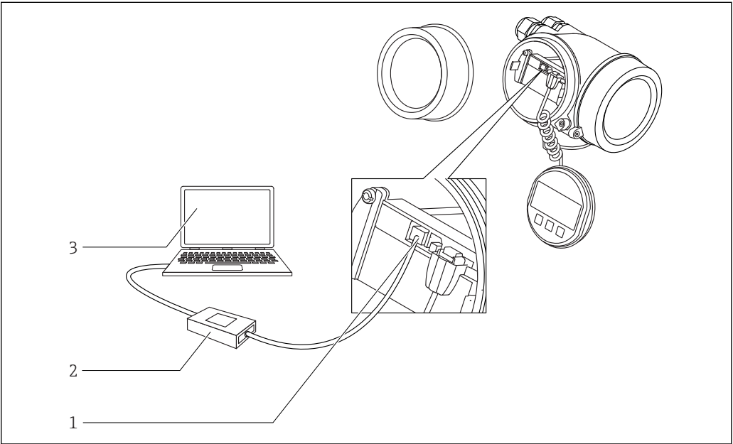
30 DeviceCare/FieldCare, 使用服务接口 (CDI)
