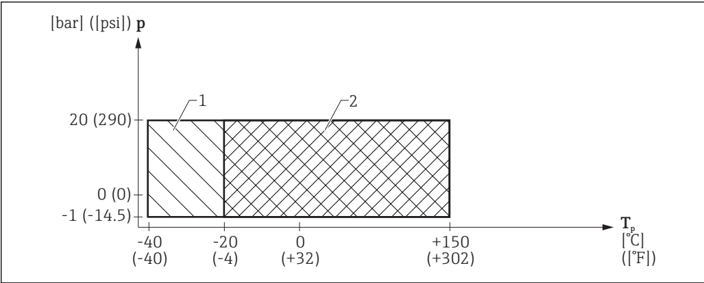
13 FMR62：允许过程温度和过程压力范围，带 PEEK 全填充一体化天线（订购选项 070，选型代号 GE、GF），150 °C (302 °F)
