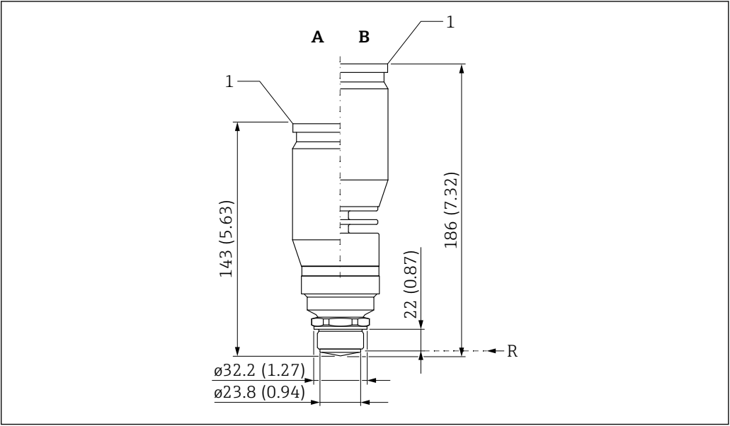
21 外形尺寸示意图; 单位: mm (in)
