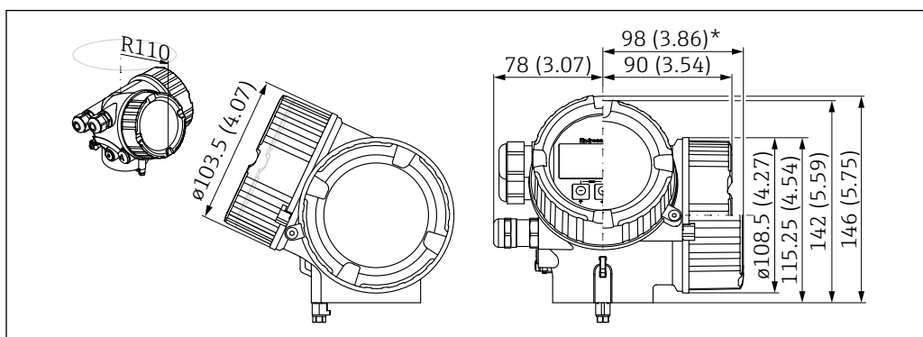
图 18 GT18 外壳 (316L) ; 单位: mm (in)
