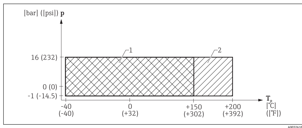
图 15 FMR62: 允许过程温度和过程压力范围, 带 Tri-Clamp 2"卡箍过程连接
