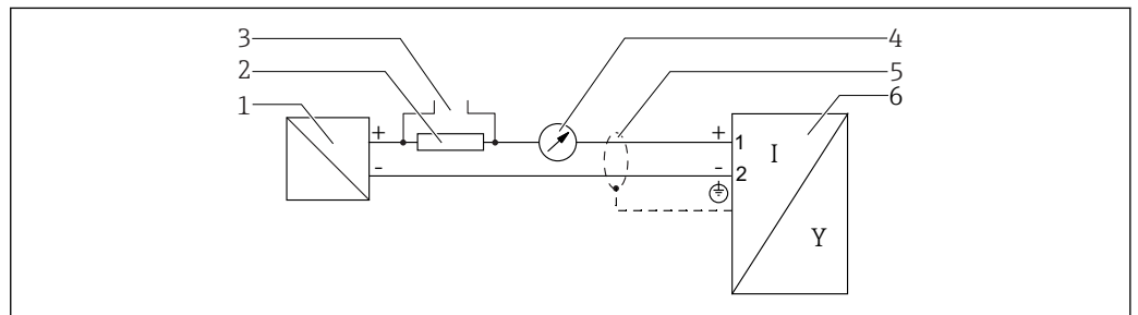
4 接线图: 两线制; 4...20 mA HART
