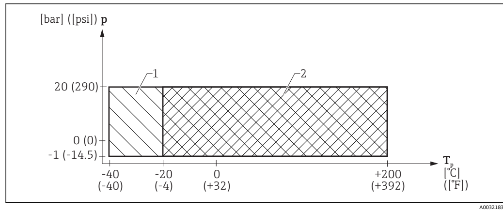
图 14 FMR62: 允许过程温度和过程压力范围, 带 PEEK 全填充一体化天线 (订购选项 070, 选型代号 GE、GF), 200 °C (392 °F)
