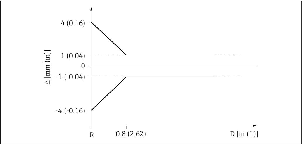
图 11 近距离测量时的最大测量误差
