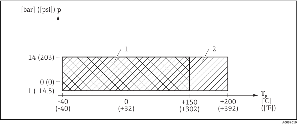
图 16 FMR62：允许过程温度和过程压力范围，带 Tri-Clamp 3"或 Tri-Clamp 4"卡箍过程连接
